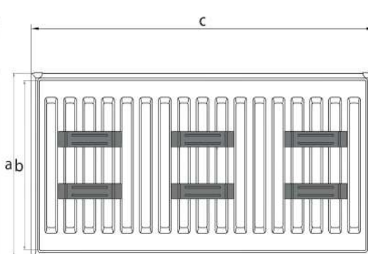
6 кронштейнов | 6 hangers; 1700/...../2000 mm
