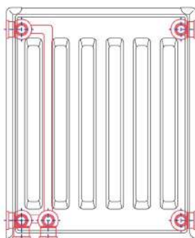
Компактное соединение на 6 отверстий с С-образным кронштейном (двойная поверхность)
