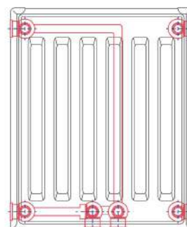
Компактное соединение на 6 отверстий с С-образным кронштейном 6 Holes Compact Middle Connection
