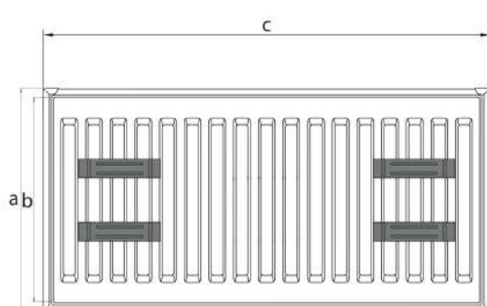
4 кронштейна | 4 hangers; 400/...../1600 mm
