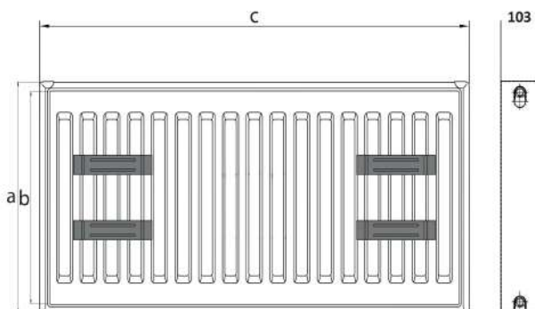
4 кронштейна | 4 hangers; 400/...../1600 mm
