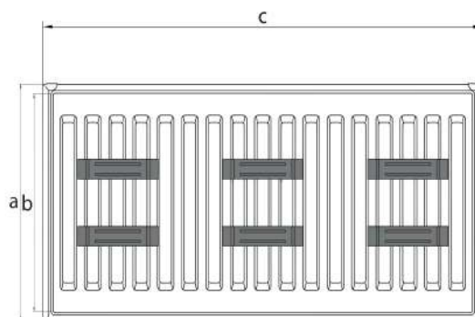
6 кронштейнов | 6 hangers; 1700/...../3000 mm
