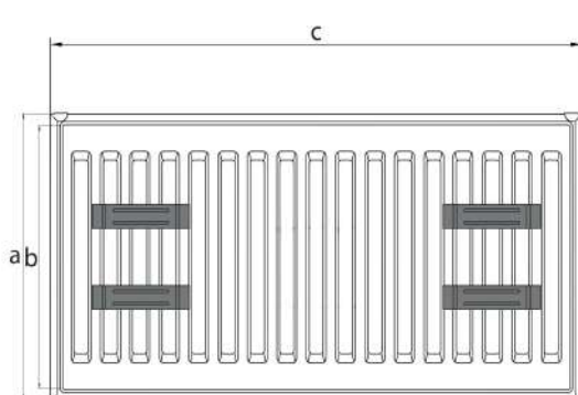
4 кронштейна | 4 hangers; 400/...../1600 mm
