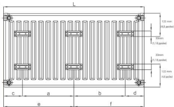
Стандартные и плоские панельные радиаторы Standard and Flat Panel Radiators
