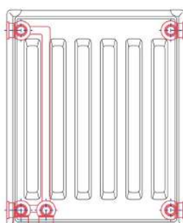
Компактное соединение на 6 отверстий с С-образным кронштейном (двойная поверхность) 6 Holes Compact Connection with C Bracket (Double Face)
