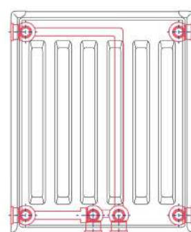
Компактное соединение на 6 отверстий с С-образным кронштейном
